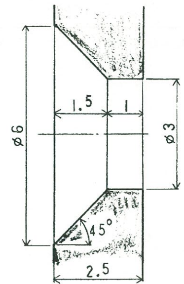
A-A 断面(1/1)
