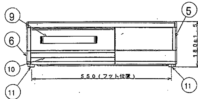
正面図
