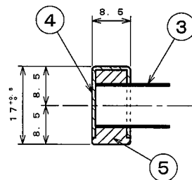
B-B断面図 S=1:1
